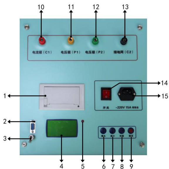
面板示意图
