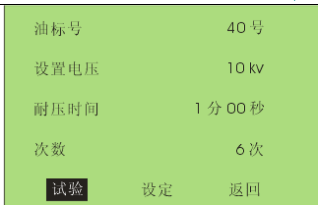
图 2.5 耐压试验主界面
