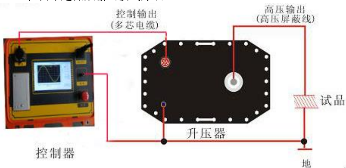
图 3 接线示意图
