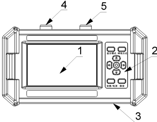
图 2-1-1 主机
