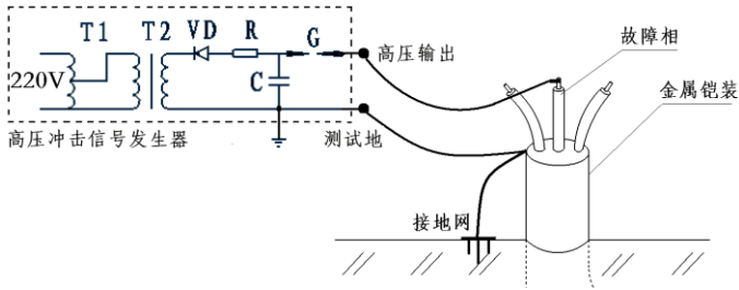
图 4-2-1 相对铠接法
