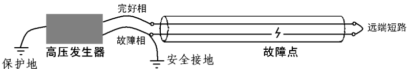
图 4-2-3 断线故障接线示意图
