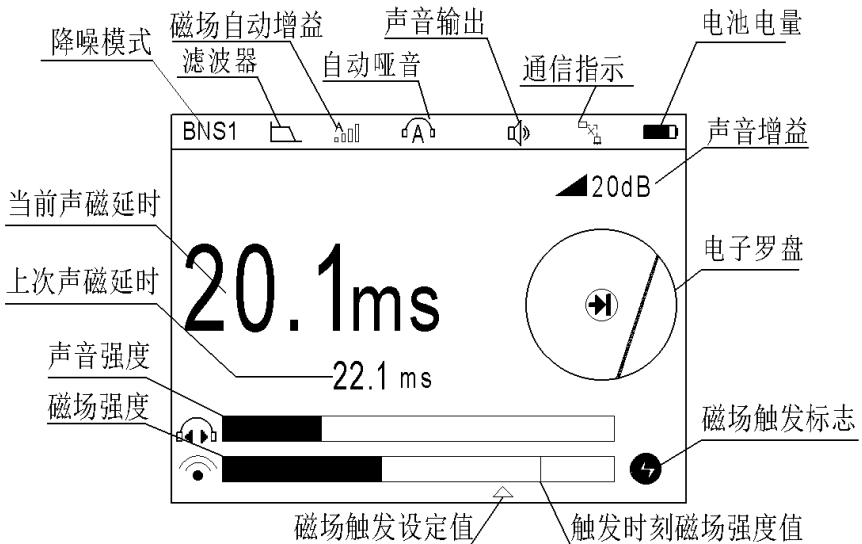
图 3-1-1 智能定点界面
