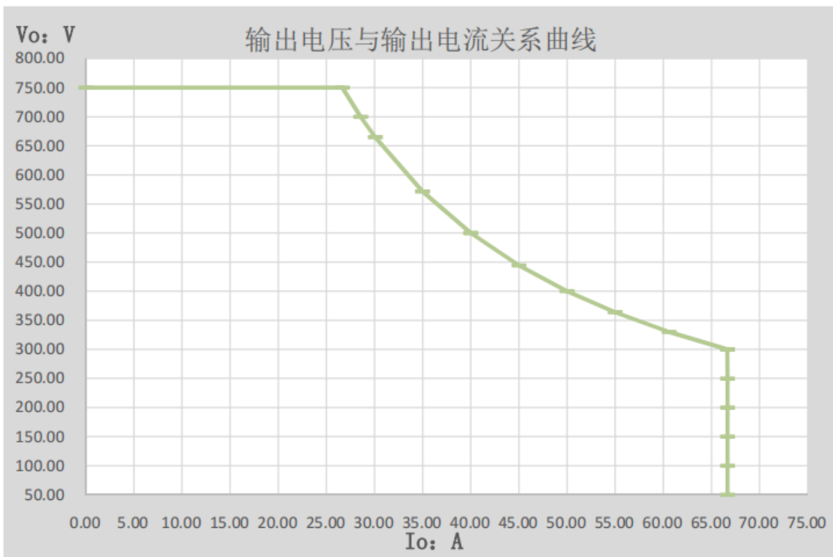
(充电电压与电流关系)
