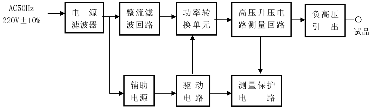
NEPRI-ZGF-B系列直流高压发生器电路框图
