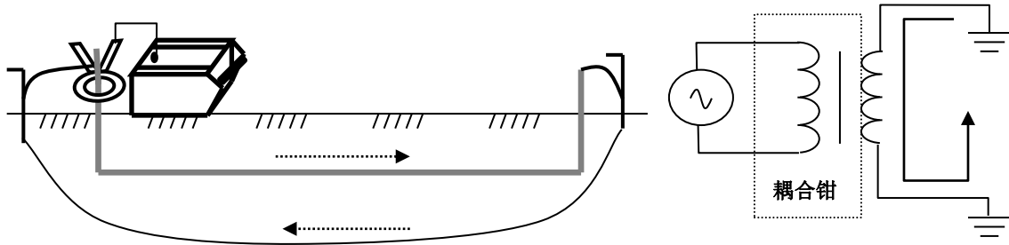
耦合法接线—示意图
