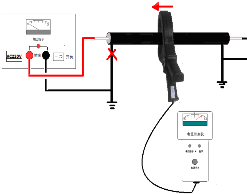
测试步骤二 测试前仪器接线
