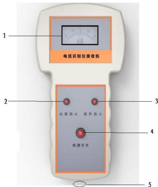
图 3-2 电缆识别仪接收机面板图
