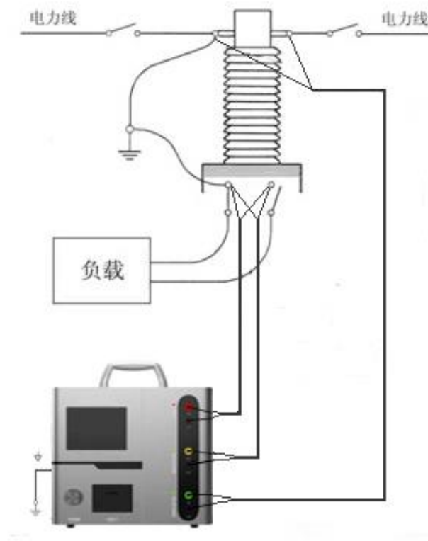
图 C.1 典型接线方式
