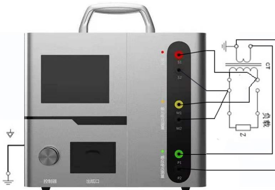
图 2.1 CT 直阻、励磁、变比试验接线方式
