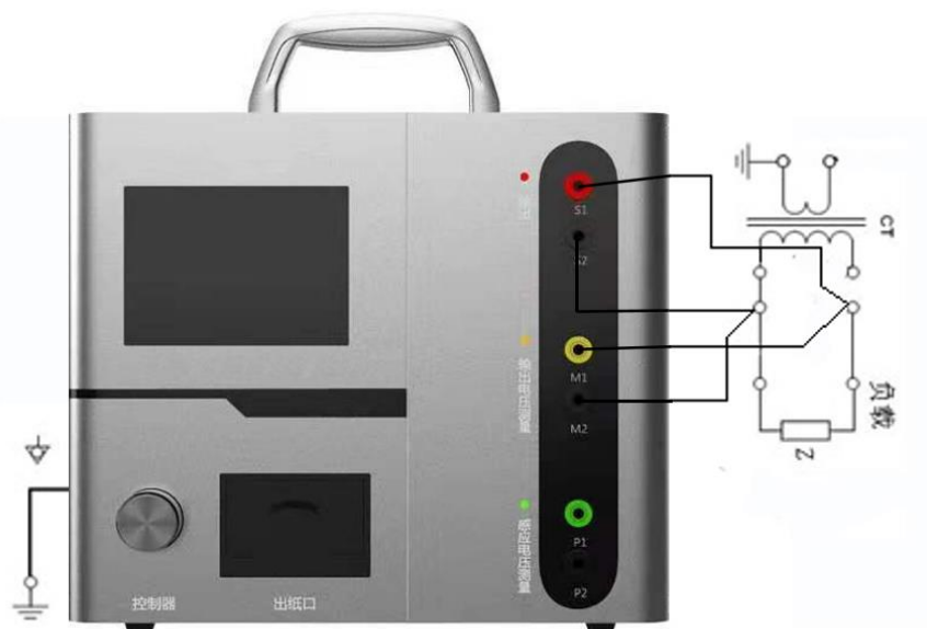
图 2.2 CT 二次负荷试验接线方式
