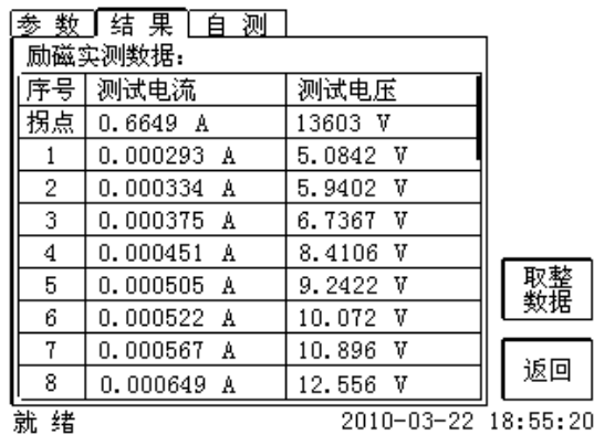
图 2.18 励磁数据界面
